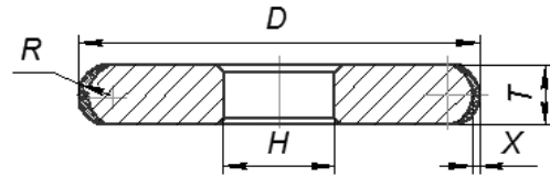
Профиль 1FF1
