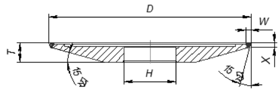
Профиль 4V9
