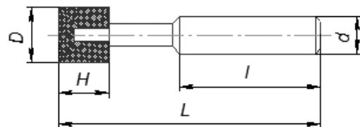
Профиль AGZ
