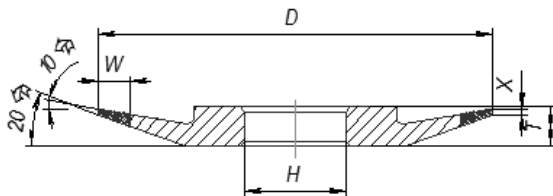
Профиль 4ВТ9
