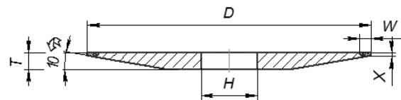
Профиль 4ЕТ9
