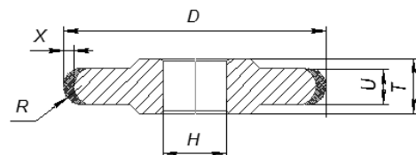
Профиль 14FF1
