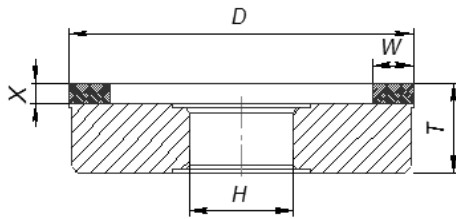
Профиль 1A2
