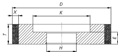
Профиль 6А1
