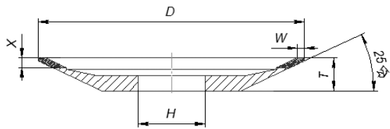
Профиль 12R4
