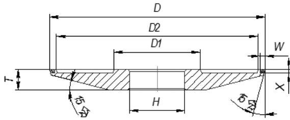
Профиль 4В9
