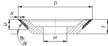
Профиль 12V9
