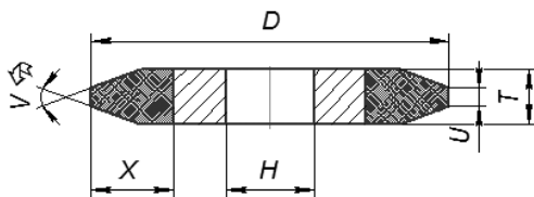
Профиль 1D1
