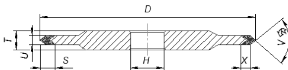
Профиль 14EE1
