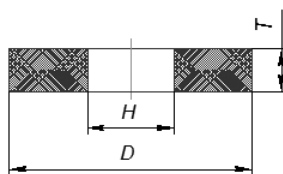
Профиль A8
